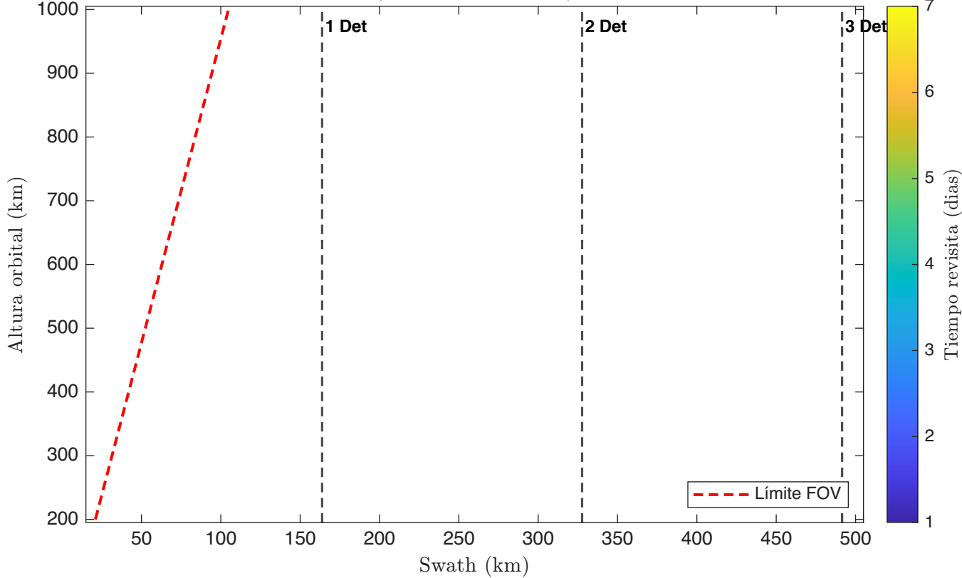
Tiempo Revisita - 1 Satellite(s); 2 Telescopio(s): Korsch; Detector 2 (Blanco: \geq 7 dias)
